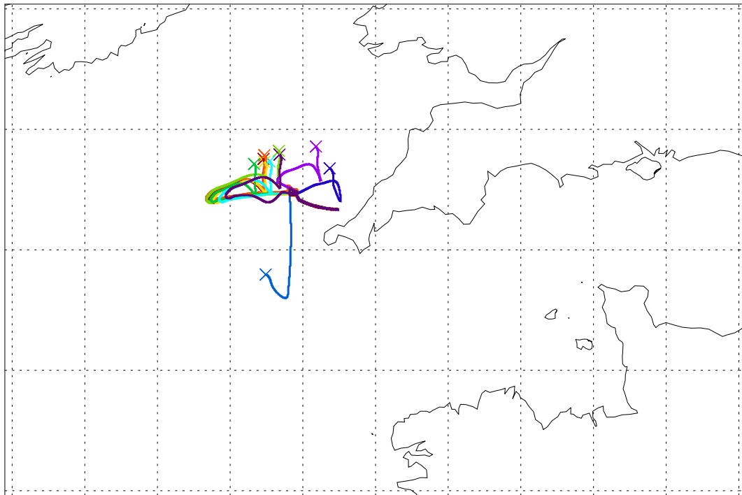
Balloon launch 04UT 04/09/2003 016hr met forecast
