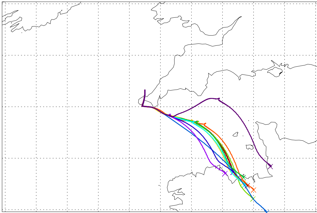
Balloon launch 04UT 12/09/2003 016hr met forecast
