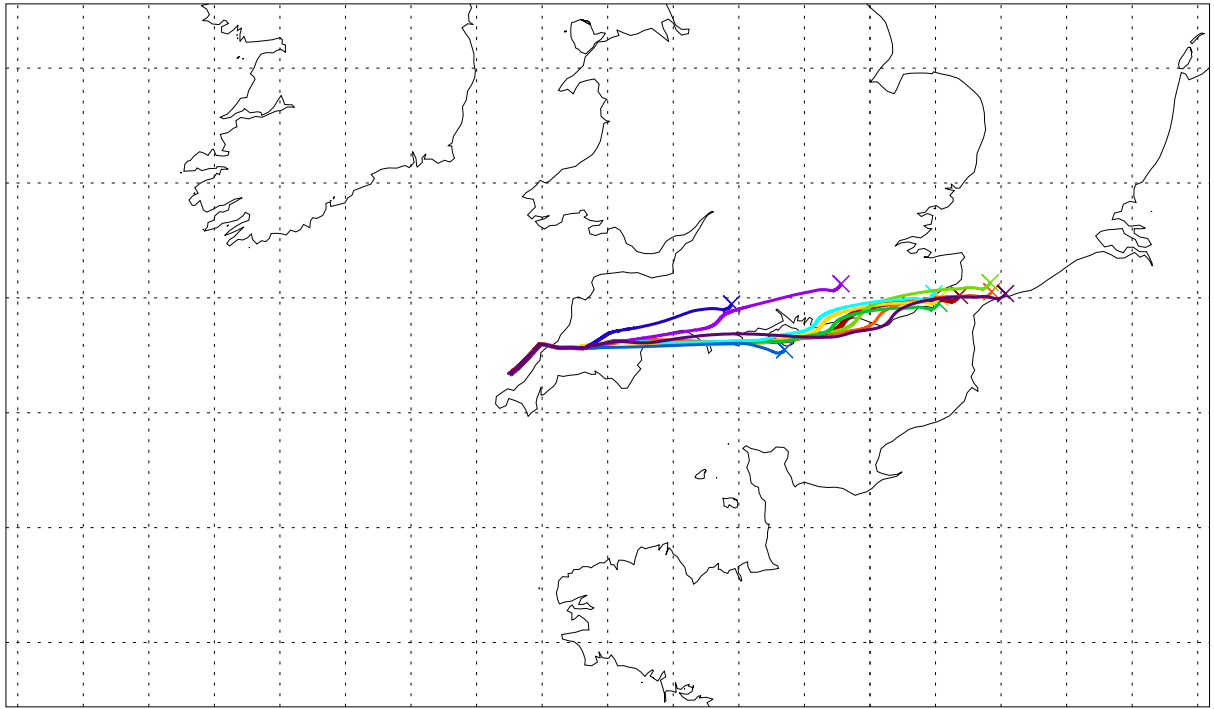
Balloon launch 04UT 29/09/2003 016hr met forecast
