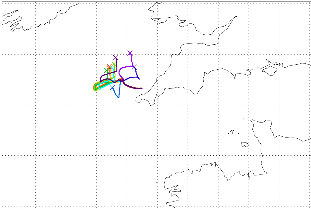
Balloon launch 04UT 04/09/2003 040hr met forecast
