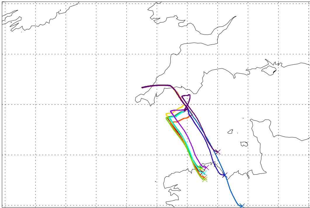
Balloon launch 04UT 10/09/2003 040hr met forecast
