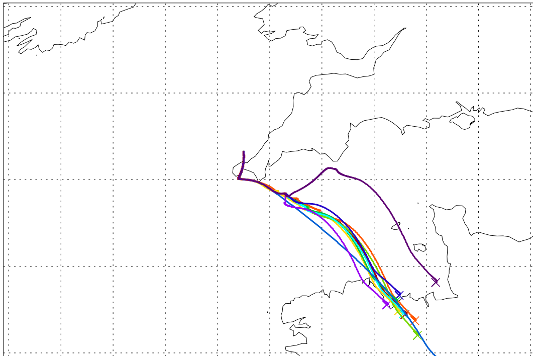
Balloon launch 04UT 12/09/2003 040hr met forecast
