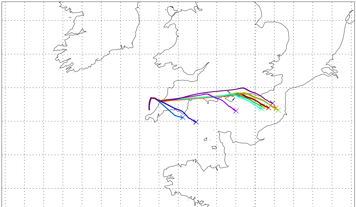
Balloon launch 04UT 26/09/2003 040hr met forecast
