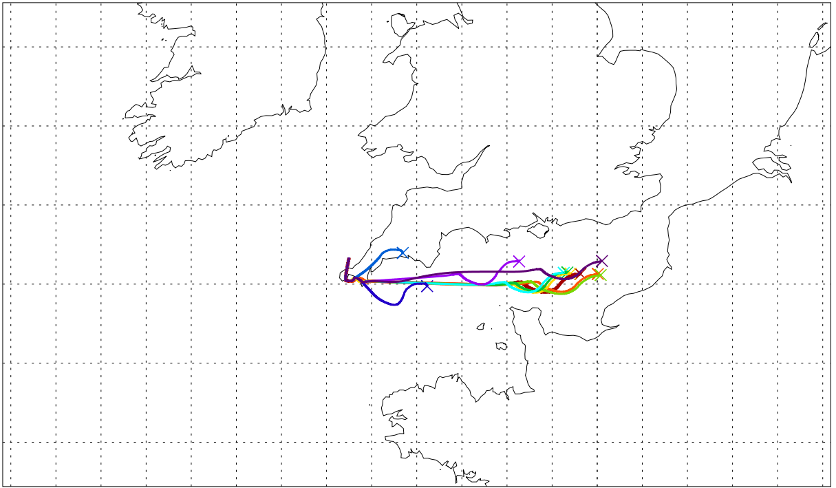
Balloon launch 04UT 27/09/2003 040hr met forecast
