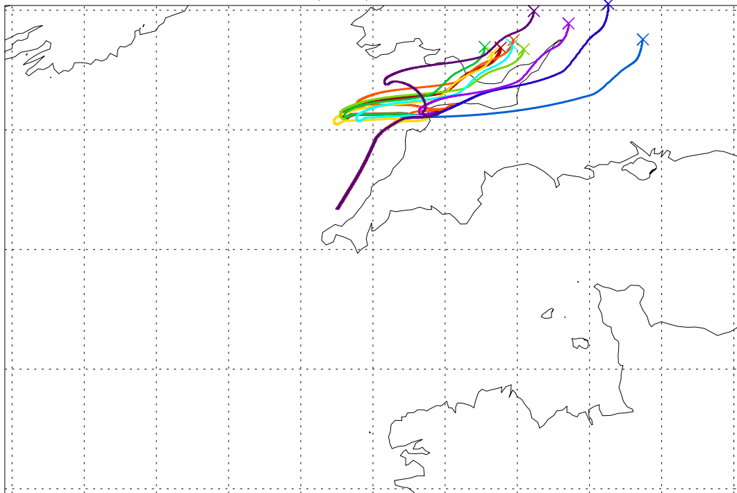
Balloon launch 04UT 07/09/2003 064hr met forecast
