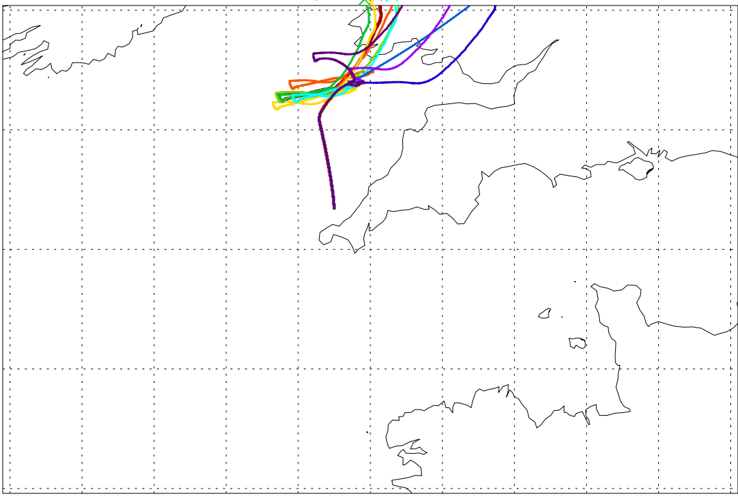
Balloon launch 04UT 07/09/2003 088hr met forecast
