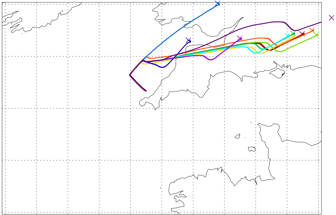
Balloon launch 04UT 20/09/2003 088hr met forecast
