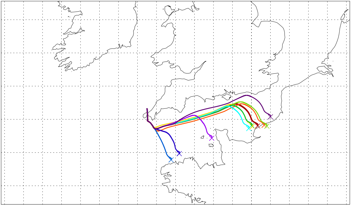
Balloon launch 04UT 23/09/2003 088hr met forecast
