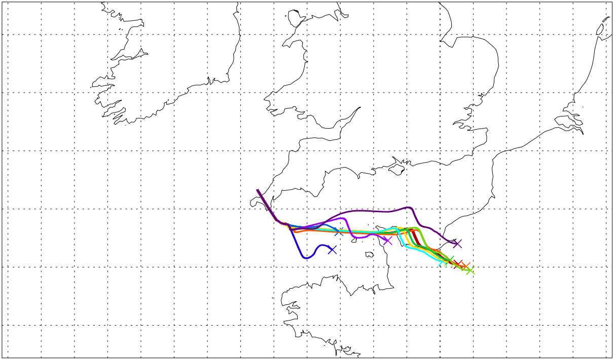
Balloon launch 04UT 27/09/2003 088hr met forecast
