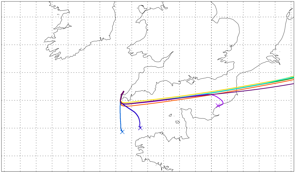
Balloon launch 04UT 25/10/2003 088hr met forecast
